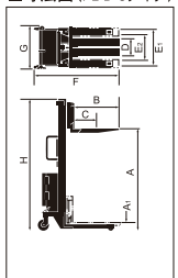
■寸法図 (PL-D-Sタイプ)
