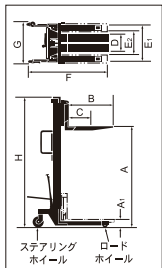
■寸法図 (PL-H-Sタイプ)
