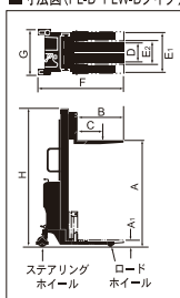
■寸法図 (PL-D・PLW-Dタイプ)
