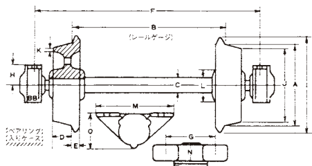
(A) 外メタルベアリング式 (標準型)
