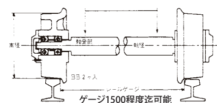
(C) ボス内ベアリング式 (急カーブのある所に適当)
