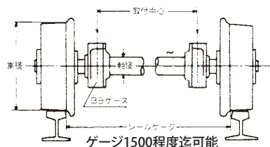
(B) 内メタルベアリング式
