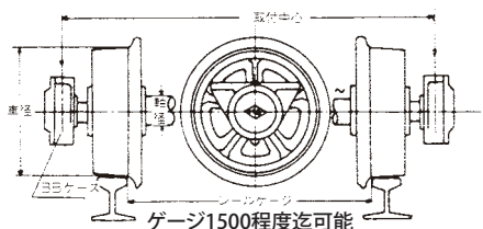
(A) 外メタルベアリング式 (標準型)
