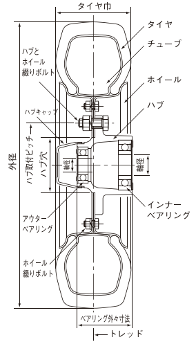
●ハブ付タイヤの構造
