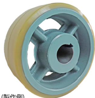
UHA200x90 40φH7 キー12x3.3
