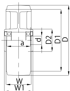
UHB200x90
