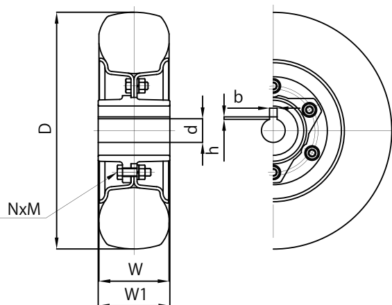
ALA3.50-5 25φH7 キー 8x3.3 ホワイトタイヤ仕様
