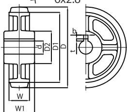
SAA150 20φH7 キー 6x2.8
