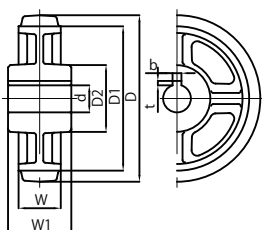
USA200 30φH7 キー 8x3.3
