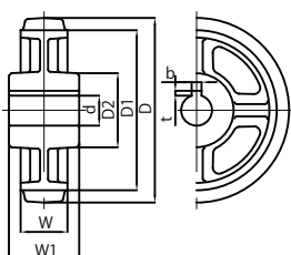
SBA150 30φH7 キー 8x3.3
