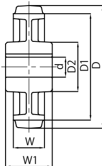
HA300x100 30φH7 キー 8x3.3
