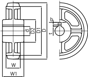
GSA A300 30φH7 キー 8x3.3
