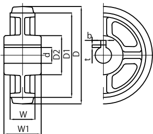
SAA150 20φH7 キー 6x2.8
