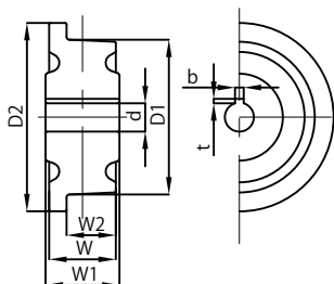
YTAA100 20φH7 キー 6x2.8
