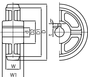
SBA150 30φH7 キー 8x3.3
