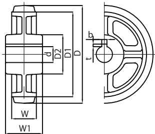
UHA200x90 40 φH7 キー 12x3.3
