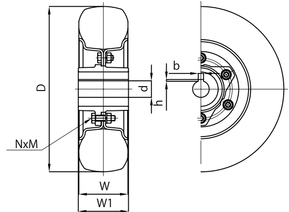
ALA3.50-5 25φH7 キー 8x3.3 ホワイトタイヤ仕様
