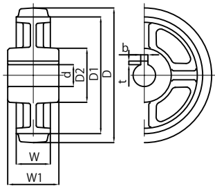
HA300x100 30φH7 キー 8x3.3
