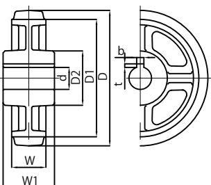
GSA150 30φH7 キー 8x3.3
