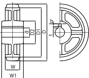
USA200 30φH7 キー 8x3.3
