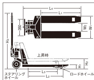
■寸法図 (標準タイプ)
